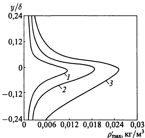
Рис. 5.61. Профили флуктуаций плотности в поперечном сечении слоя смешения при x/L = 0,25 (1); 0,5 (2); 0,75 (3)
