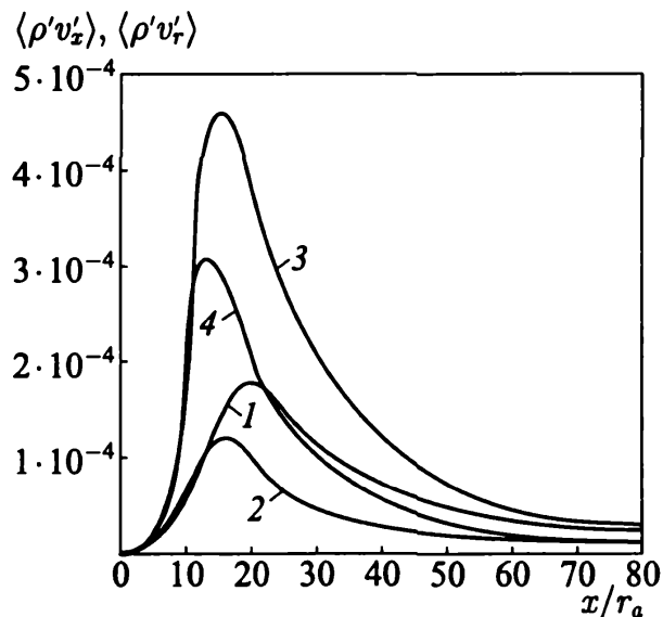
Рис. 5.40. Распределения корреляционных моментов \langle \rho'v_x' \rangle (кривые 1, 3) и \langle \rho'v_r' \rangle (кривые 2, 4) вдоль оси струи при \vartheta = 0,6 (кривые 1, 2) и \vartheta = 2 (кривые 3, 4)
