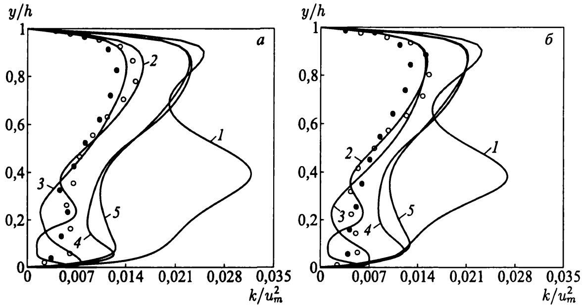
Рис. 5.18. Распределения кинетической энергии турбулентности при x/h = 40 (фрагмент а) и x/h = 50 (фрагмент б)
