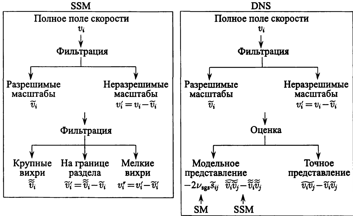
Рис. 3.4. Разрешимые и неразрешимые масштабы в модели подобных масштабов
