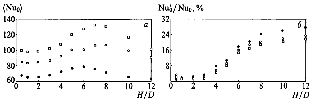
Рис. 5.56. Зависимость среднего числа Нуссельта (фрагмент a ) и его флуктуаций (фрагмент б ) от расстояния до преграды при Re = 10^4 (значки \bullet ); 2 \cdot 10^4 (значки \circ ); 3 \cdot 10^4 (значки \square )
