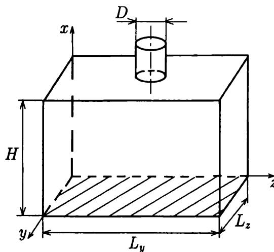
Рис. 5.43. Расчетная область и система координат
