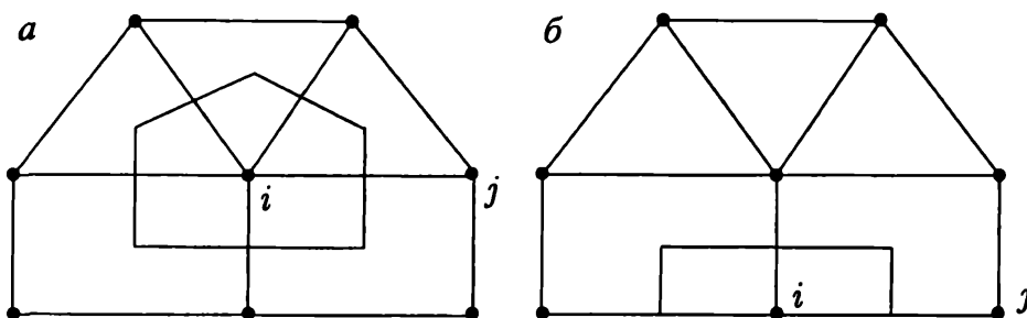
Рис. 4.5. Внутренний (фрагмент а) и граничный (фрагмент б) контрольные объемы
