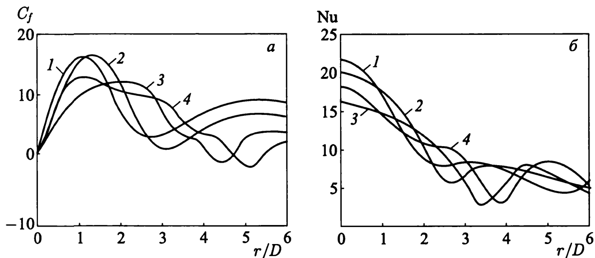
Рис. 5.53. Зависимость коэффициента трения (фрагмент a ) и числа Нуссельта (фрагмент б ) от времени при H/D = 5 и Re = 500 . Кривые соответствуют моментам времени t = 10 (1); 20 (2); 30 (3); 40 (4)
