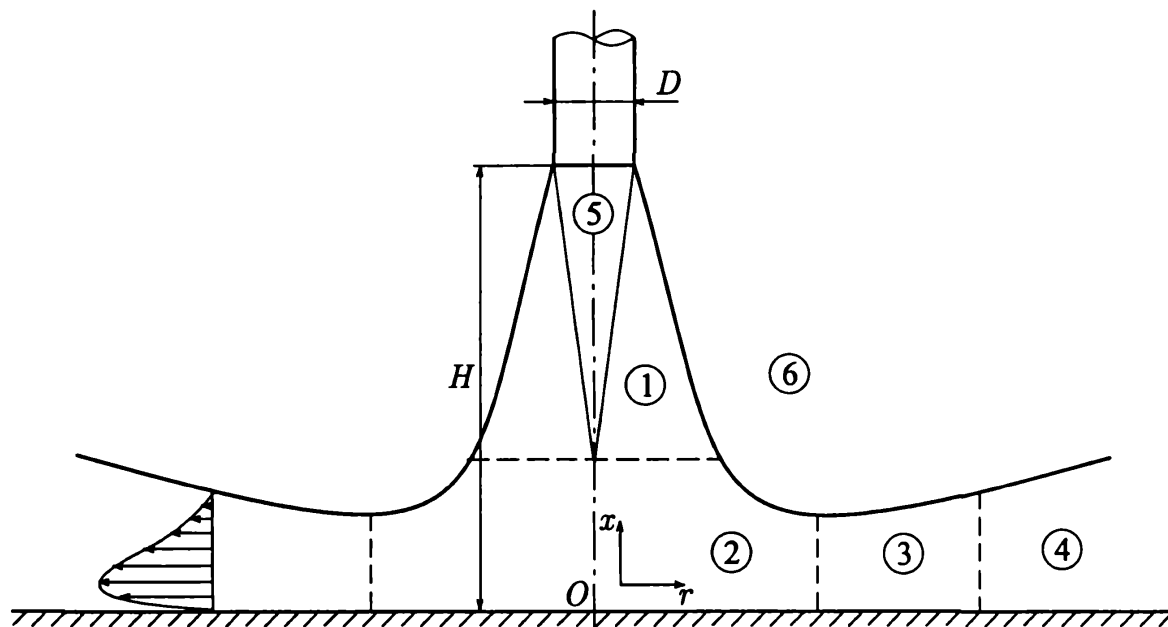
Рис. 5.42. Характерные области течения
