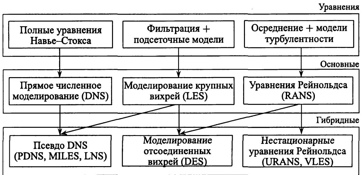
Рис. 1.4. Методы моделирования турбулентных течений
