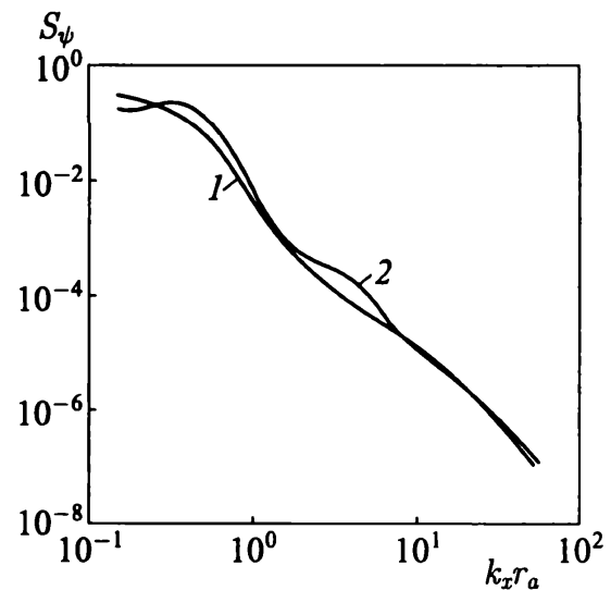
Рис. 5.64. Спектр флуктуаций фазы в круглой струе при Re = 5 \cdot 10^3 (кривая 1) и Re = 1,5 \cdot 10^4 (кривая 2)
