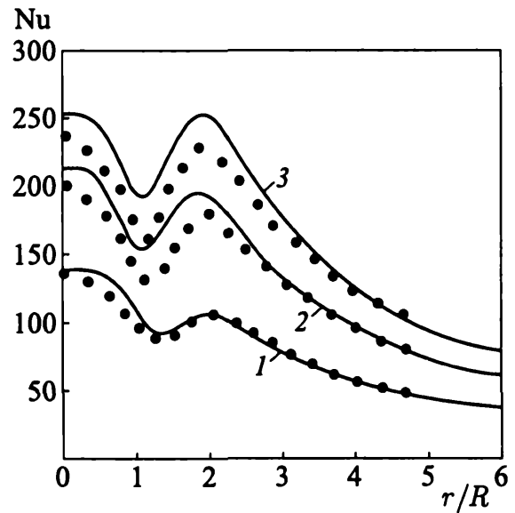
Рис. 5.49. Сравнение распределения числа Нуссельта по поверхности преграды с данными физического эксперимента [69, 124] (значки \bullet ) при H/D = 2 и Re = 2,3 \cdot 10^4 (1); 5 \cdot 10^4 (2); 7 \cdot 10^4 (3)
