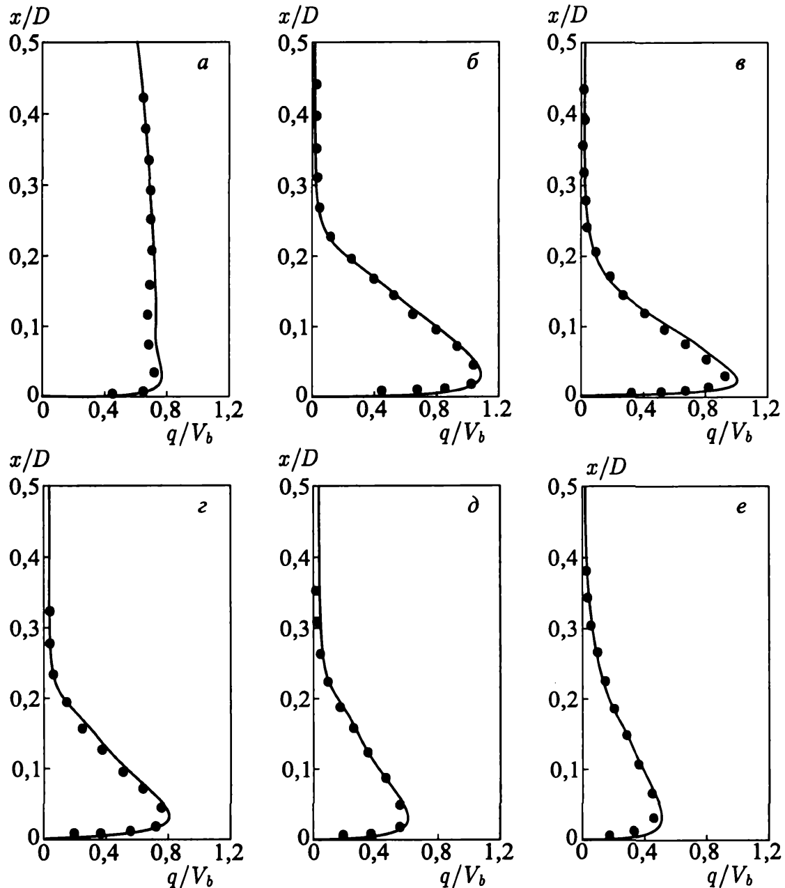
Рис. 5.44. Распределения скорости в различных сечениях по радиальной координате r/D = 0,5 (а); 1 (б); 1,5 (в); 2 (г); 2,5 (д); 3 (е) при H/D = 2 , Re = 2,3 \cdot 10^4 . Значки • соответствуют данным измерений [69, 70]
