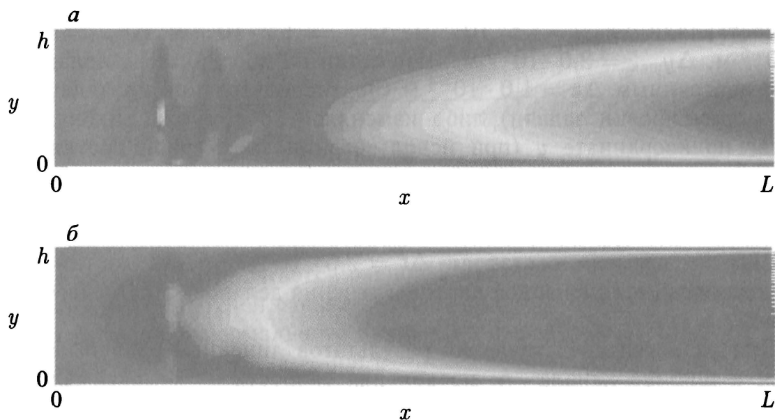
Рис. 5.11. Линии уровня продольной скорости при v_{w1} = 0 м/с, v_{w2} = 2,75 м/с (фрагмент а) и v_{w1} = 2,75 м/с, v_{w2} = 2,75 м/с (фрагмент б)
