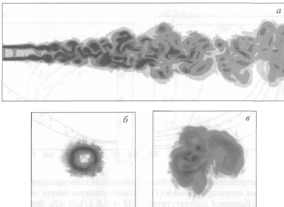
Рис. 5.32. Линии уровня вихря скорости в момент времени t = 2,32 с в срединном сечении (фрагмент a ) и сечениях x/r_a = 10 (фрагмент б ) и x/r_a = 80 (фрагмент в )
