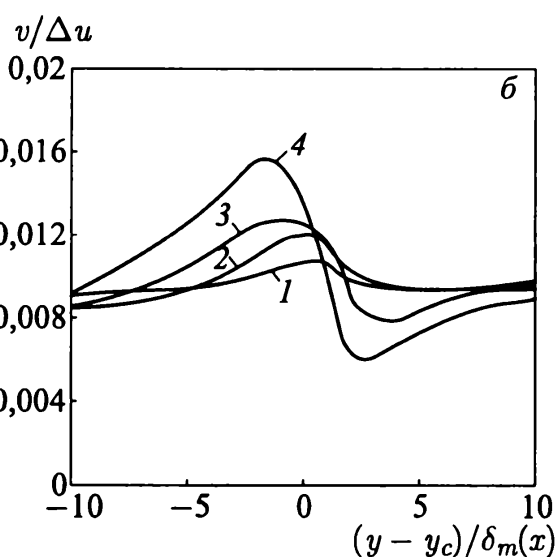
Рис. 5.26. Профили продольной (фрагмент а) и поперечной (фрагмент б) скорости при M_c = 0,2 (1); 0,4 (2); 0,6 (3); 0,8 (4). Значки \bullet соответствуют расчетным данным [148]
