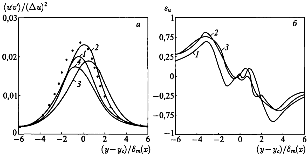
Рис. 5.29. Распределения сдвиговых напряжений (фрагмент а) и коэффициента асимметрии (фрагмент б) в сравнении с экспериментальными данными [169] (значки \bullet ) при x/L_x = 0,6 (1); 0,7 (2); 0,8 (3); 0,9 (4)
