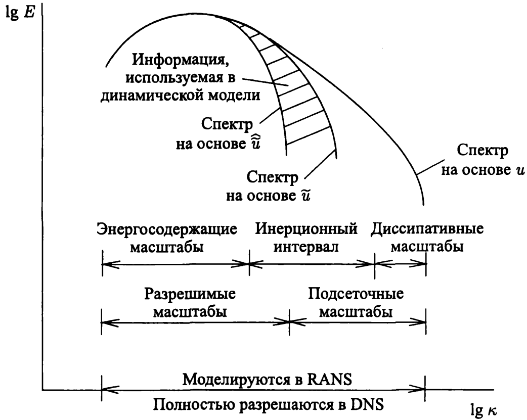
Рис. 3.3. Волновые спектры, построенные на основе мгновенной, фильтрованной и дважды фильтрованной скорости
