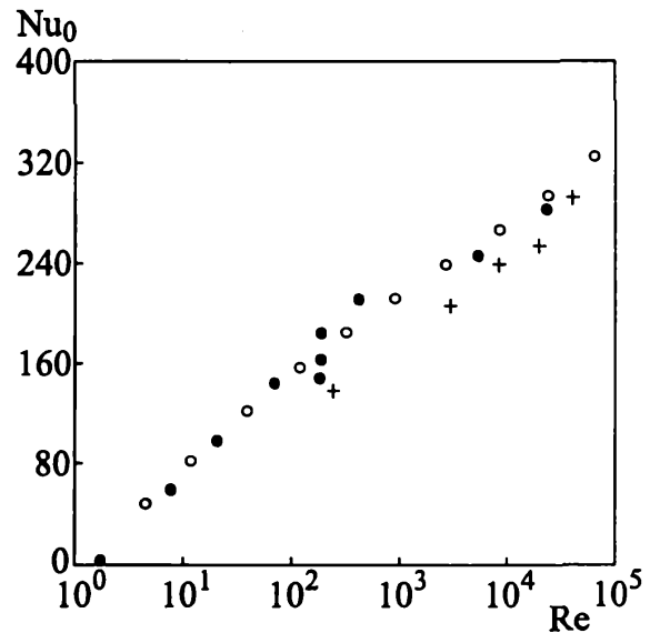
Рис. 5.51. Зависимость числа Нуссельта в точке торможения от числа Рейнольдса при H/D = 6,0 . Значки \circ соответствуют результатам расчета, значки \bullet — данным [69, 124], + — расчету по SST-модели [328]
