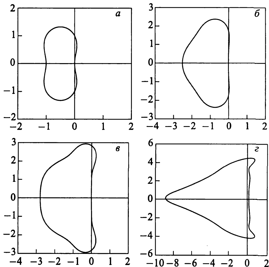
Рис. 4.8. Области устойчивости методов Рунге–Кутты порядка k = 2 (а); 3 (б); 4 (в); 5 (г)
