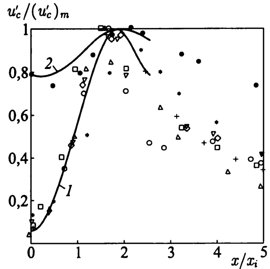
Рис. 5.36. Распределения интенсивности турбулентности вдоль осевой координаты
