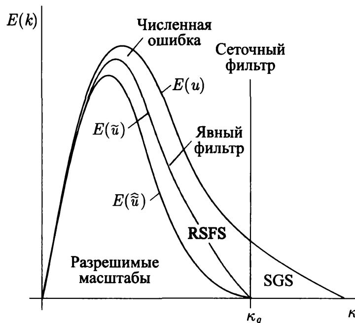
Рис. 3.6. Разрешимые и неразрешимые масштабы турбулентного движения при использовании явной фильтрации
