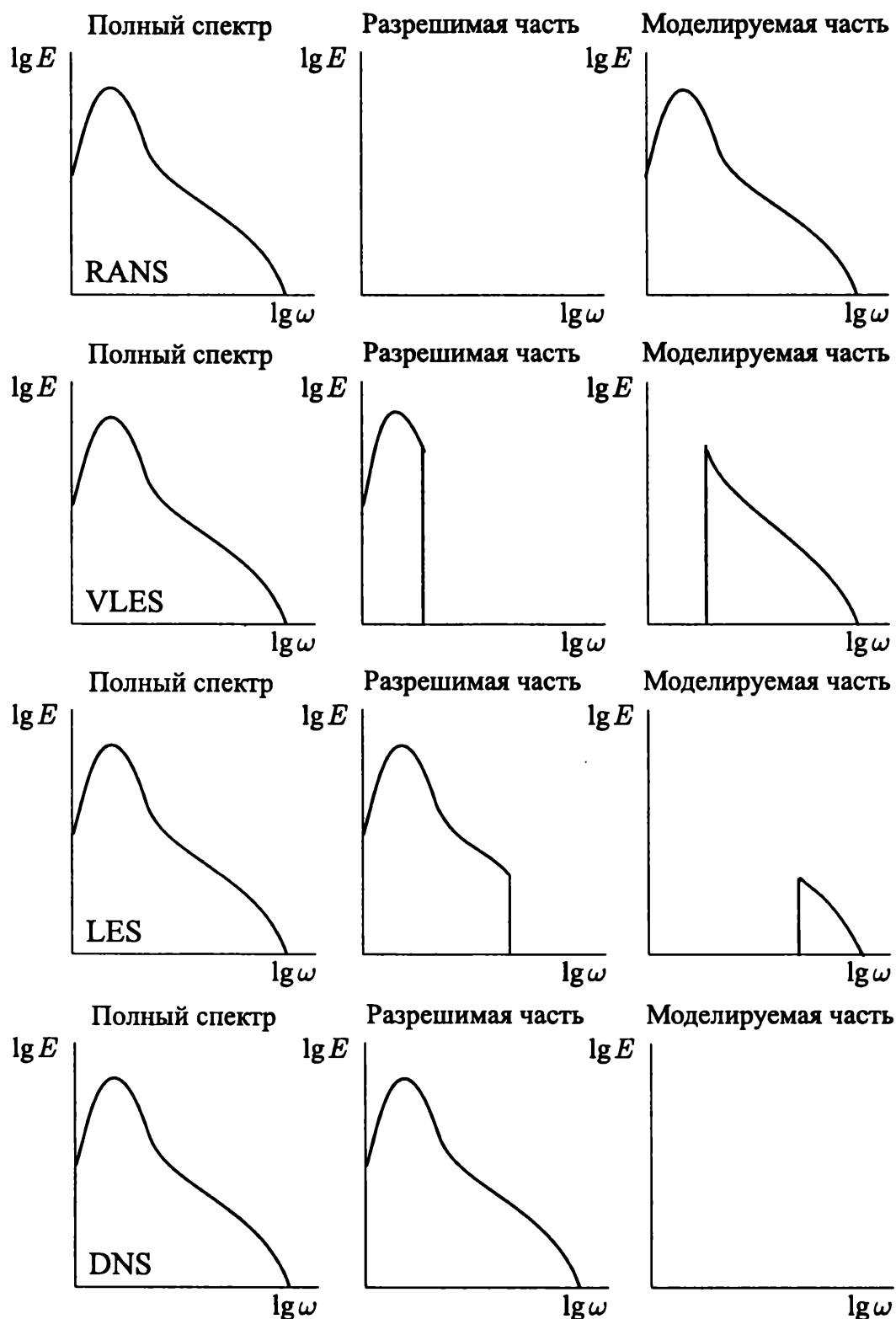
Рис. 1.6. Соотношения между разрешимой и моделируемой частями спектра турбулентности
