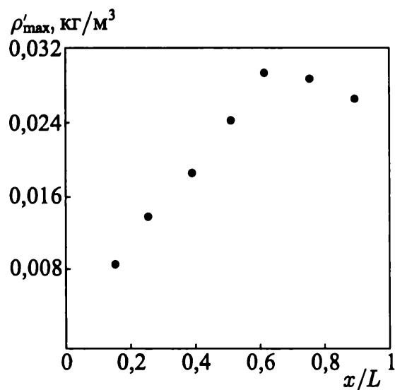
Рис. 5.62. Зависимость максимального уровня флуктуаций плотности от продольной координаты в слое смешения
