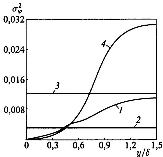
Рис. 5.60. Распределения дисперсии флуктуаций фазовой функции волнового фронта в пограничном слое. Кривая 1 соответствует результатам расчета, 2 — расчету по (5.4) при A = 0,1 , 3 — расчету по (5.4) при A = 0,2 , 4 — расчету по (5.5)
