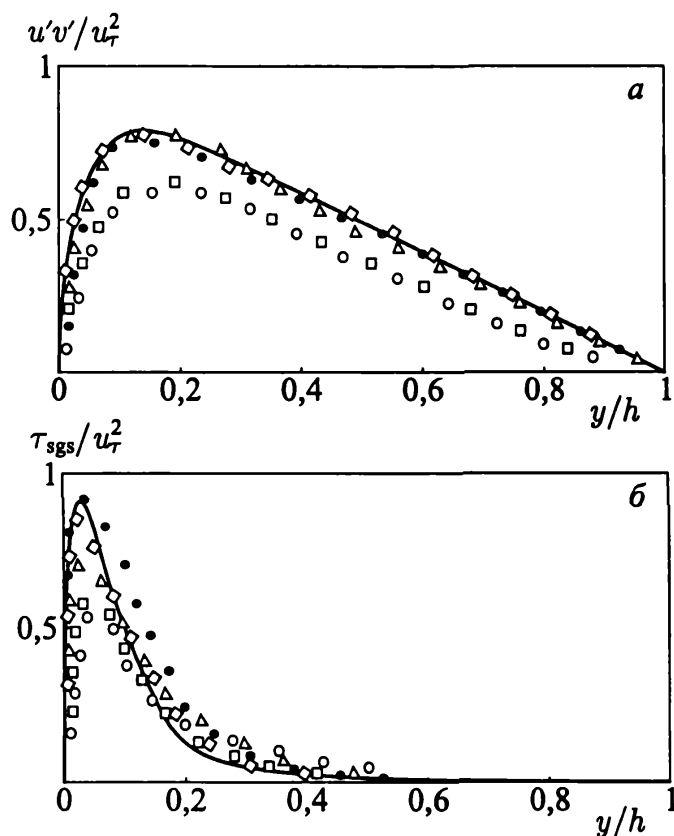
Рис. 5.6. Распределения рейнольдсовых (фрагмент а) и подсеточных напряжений (фрагмент б)
