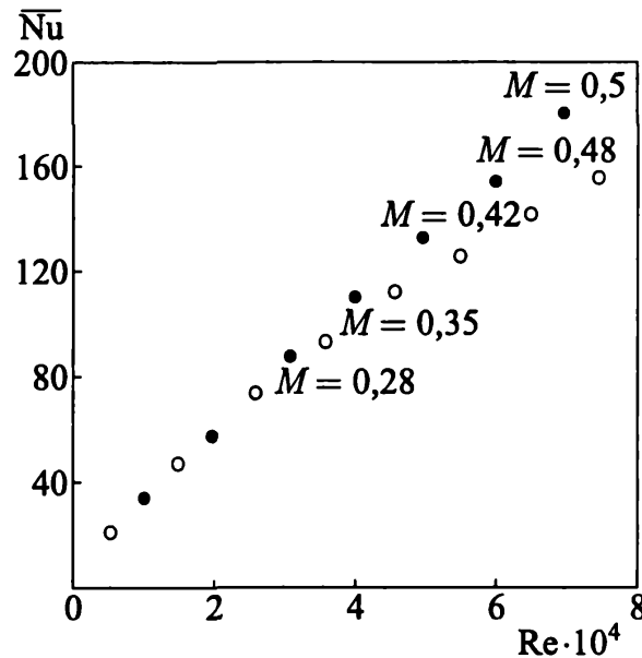
Рис. 5.57. Зависимость среднего числа Нуссельта от числа Маха. Значки \bullet соответствуют расчетным данным для сжимаемой жидкости, а значки \circ — несжимаемой жидкости
