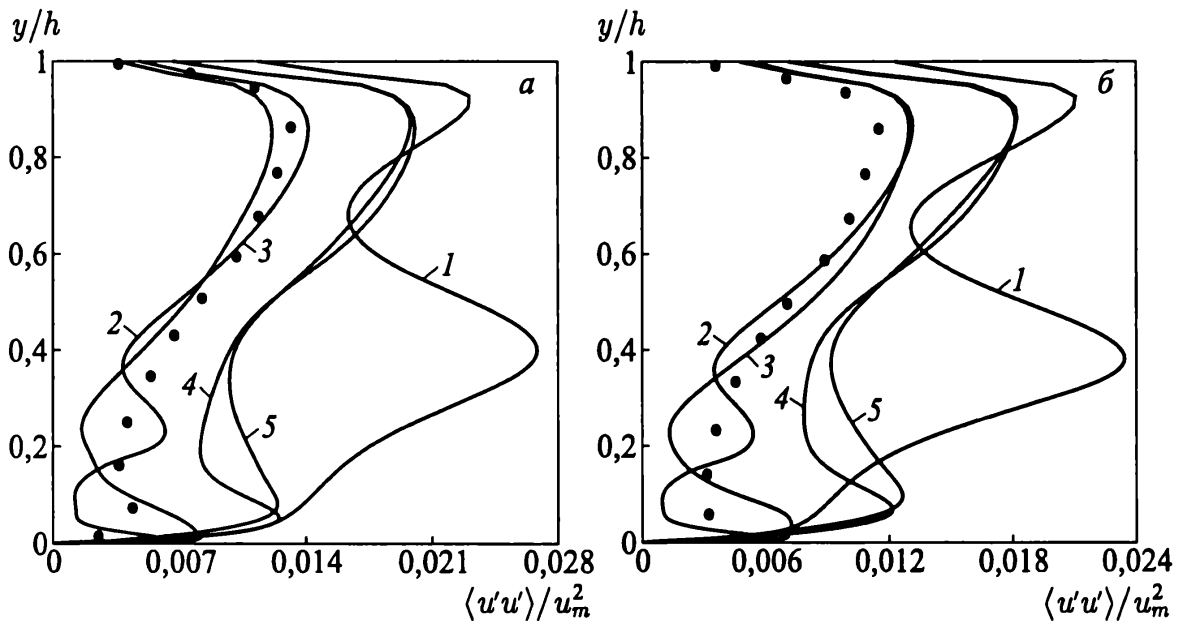
Рис. 5.20. Распределения рейнольдсовых напряжений \langle u'u' \rangle при x/h = 40 (фрагмент а) и x/h = 50 (фрагмент б)
