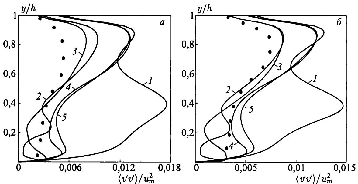
Рис. 5.22. Распределения рейнольдсовых напряжений \langle v'v' \rangle при x/h = 40 (фрагмент а) и x/h = 50 (фрагмент б)
