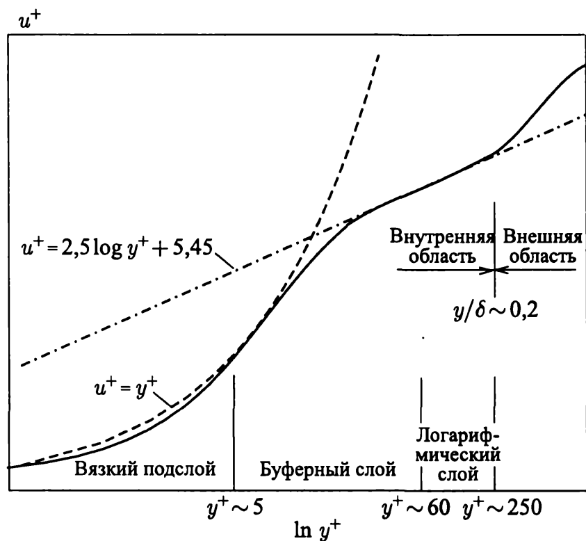
Рис. 4.12. Структура пограничного слоя
