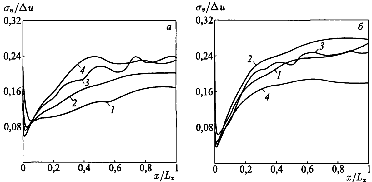
Рис. 5.30. Распределения максимального уровня пульсаций продольной (фрагмент а) и поперечной (фрагмент б) скорости вдоль координаты x при M_c = 0,2 (1); 0,4 (2); 0,6 (3); 0,8 (4)
