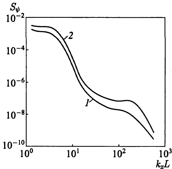
Рис. 5.63. Спектр флуктуаций фазы в свободном слое смешения при M_c = 0,2 (кривая 1) и M_c = 0,8 (кривая 2)
