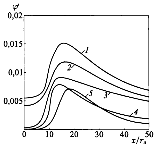
Рис. 5.37. Распределения среднеквадратических значений пульсаций скорости, температуры и смешанного корреляционного момента пульсаций скорости и температуры вдоль оси струи при \vartheta = 1,2
