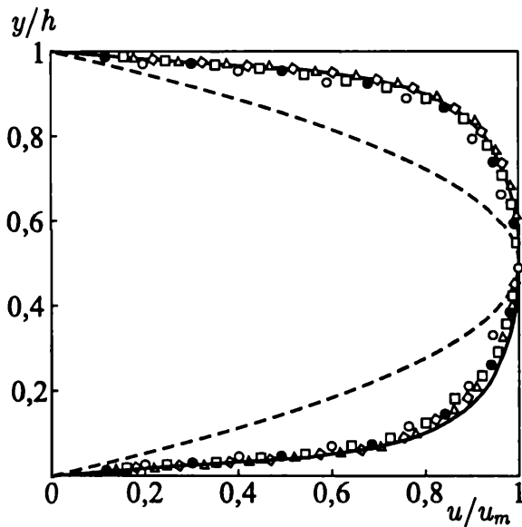
Рис. 5.2. Распределения продольной скорости в поперечном сечении
