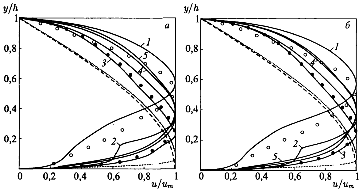
Рис. 5.13. Распределения продольной скорости при x/h = 40 (фрагмент а) и x/h = 50 (фрагмент б)
