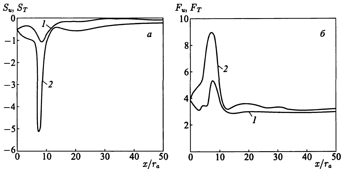
Рис. 5.41. Распределения коэффициентов асимметрии (фрагмент а ) и эксцесса (фрагмент б ) пульсаций скорости (кривые 1) и температуры (кривые 2) вдоль оси струи при \vartheta = 1,2
