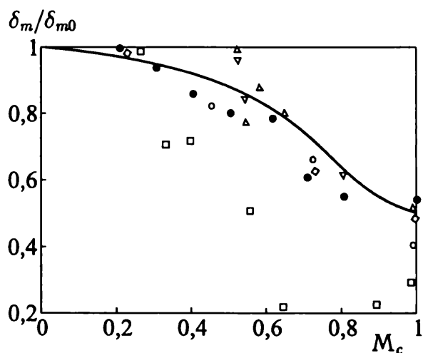
Рис. 5.31. Зависимость толщины потери импульса от числа Маха. Значки ● соответствуют результатам расчета, □ — [262], △, ▽, ◇ — [148], ○ — [169]
