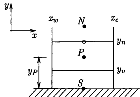
Рис. 4.14. Пристеночный контрольный объем
