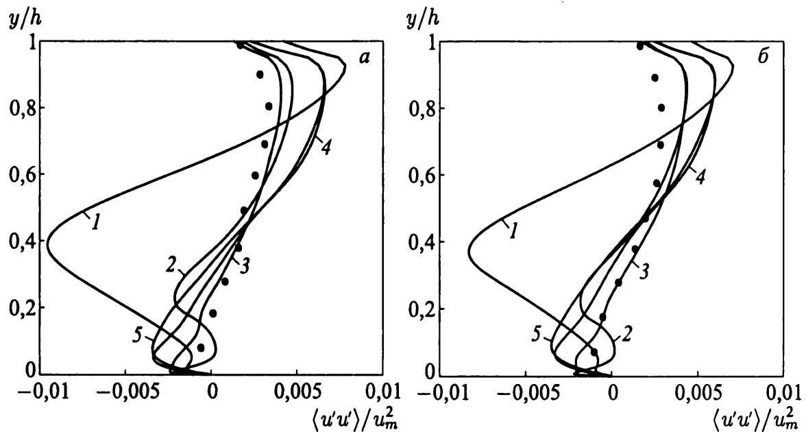
Рис. 5.21. Распределения рейнольдсовых напряжений \langle u'v' \rangle при x/h = 40 (фрагмент а) и x/h = 50 (фрагмент б)
