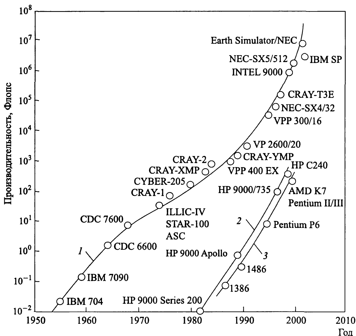
Рис. 4.2. Динамика увеличения производительности вычислительных систем различного класса (1 — суперкомпьютеры; 2 — рабочие станции; 3 — персональные компьютеры)
