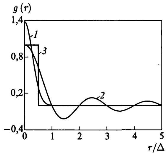
Рис. 2.4. Преобразования Фурье, соответствующие фильтрующим функциям (1 — коробочный, 2 — гауссовский, 3 — Фурье)
