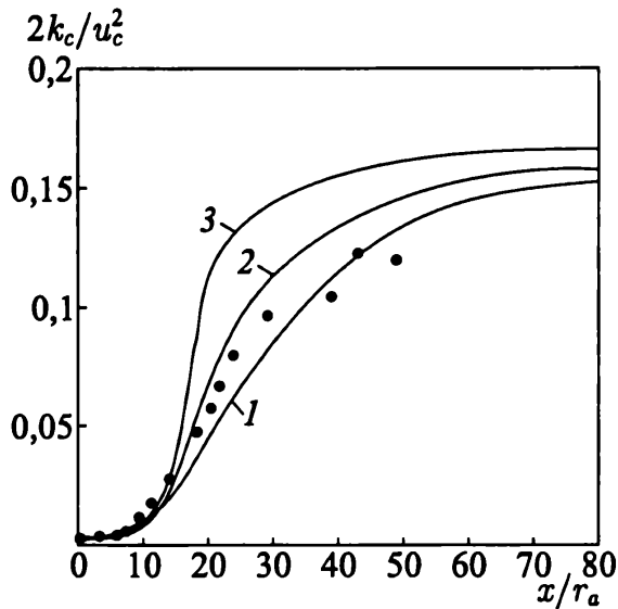
Рис. 5.35. Распределения кинетической энергии турбулентности вдоль оси струи при \vartheta = 0,6 (1); 1 (2); 2 (3). Значки • соответствуют данным [102] при \vartheta = 0,7
