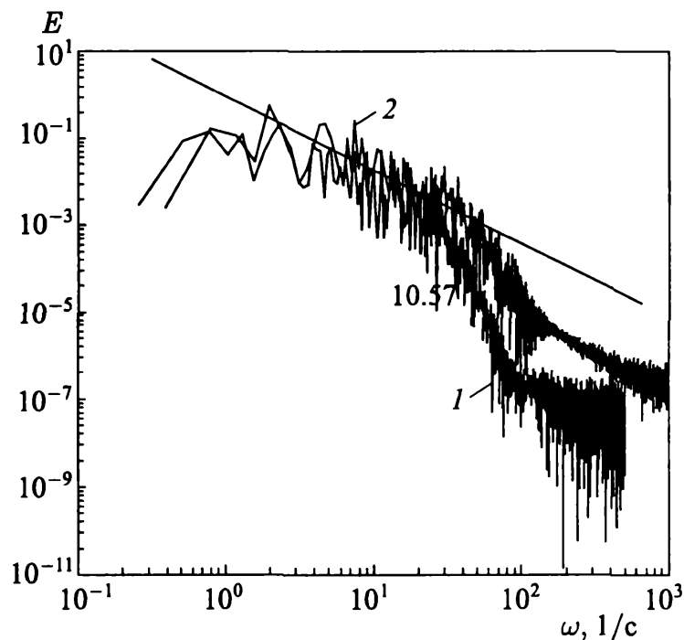
Рис. 5.10. Спектр кинетической энергии турбулентности (1 — расчет на грубой сетке 200 \times 50 \times 25 ; 2 — расчет на подробной сетке 400 \times 100 \times 50 )
