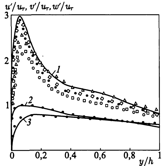
Рис. 5.5. Распределения пульсационной скорости по поперечному сечению канала (1 — u' ; 2 — v' ; 3 — w' ) при Re_\tau = 360
