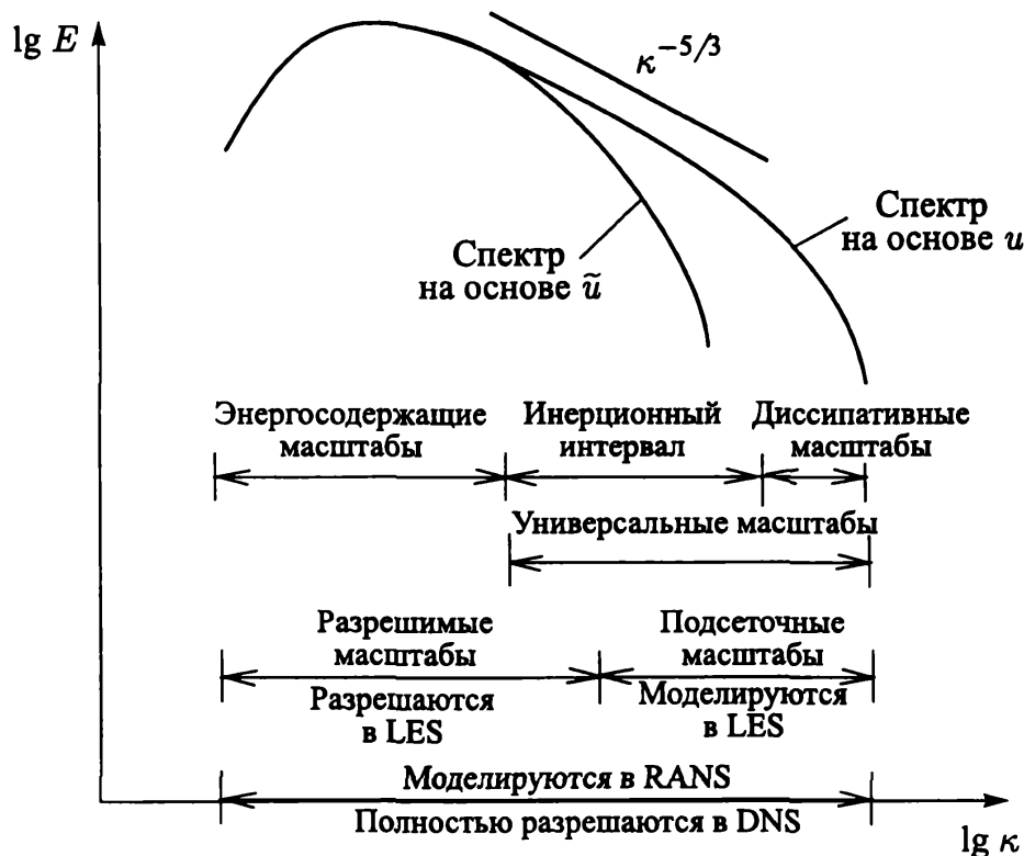
Рис. 1.9. Спектры кинетической энергии турбулентности, построенные на основе мгновенной и фильтрованной скорости
