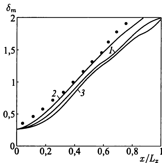
Рис. 5.25. Изменение толщины потери импульса вдоль координаты x в зависимости от формулировки граничных условий во входном сечении при \sigma_u/u_c = 0,01 (1); 0,03 (2); 0,08 (3)
