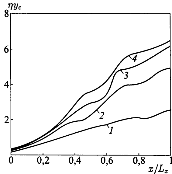
Рис. 5.27. Зависимость положения разделительной линии тока от эффективного числа Маха при M_c = 0,2 (1); 0,4 (2); 0,6 (3); 0,8 (4)
