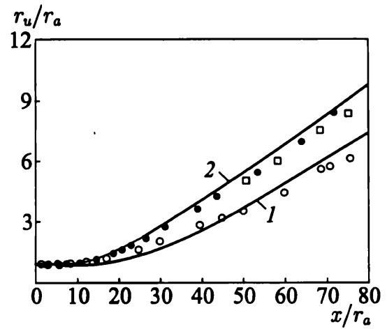
Рис. 5.34. Распределения половинного радиуса вдоль оси струи при \vartheta = 0,6 (1); 1 (2). Значки \square соответствуют данным [261] при \vartheta = 1 , значки \bullet и \circ — данным [102] при \vartheta = 0,7
