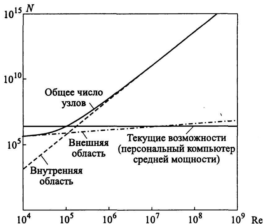
Рис. 1.10. Число узлов, необходимых для разрешения пограничного слоя
