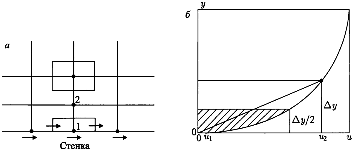
Рис. 4.13. Внутренний и граничный контрольные объемы (фрагмент а) и профиль скорости в пограничном слое (фрагмент б)
