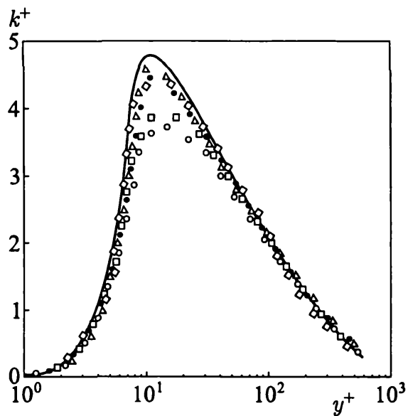
Рис. 5.4. Распределение кинетической энергии турбулентности вблизи стенки
