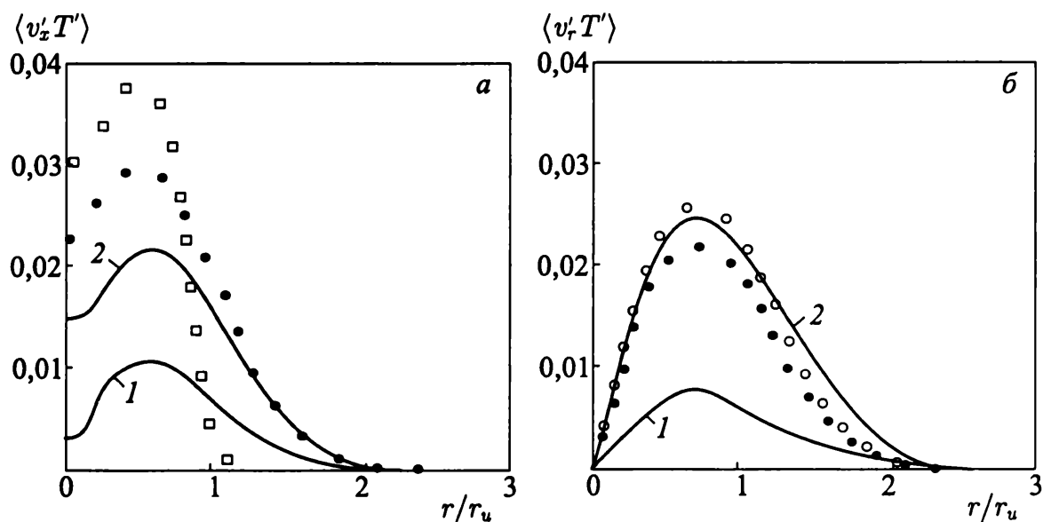
Рис. 5.38. Распределения смешанных корреляционных моментов пульсаций осевой скорости и температуры (фрагмент а) и радиальной скорости и температуры (фрагмент б) при \vartheta = 1,2 в сечениях x/r_a = 10 (кривые 1) и x/r_a = 30 (кривые 2) в сравнении с данными [58] (значки \square ), [105] (значки \bullet ), [109] (значки \circ )
