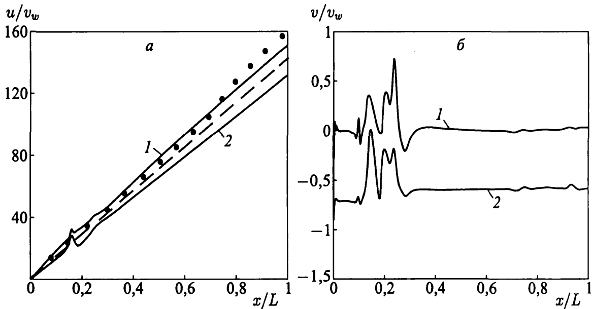
Рис. 5.15. Распределения продольной (фрагмент а) и поперечной (фрагмент б) скорости при y/h = 0,5 (1); 0,75 (2)
