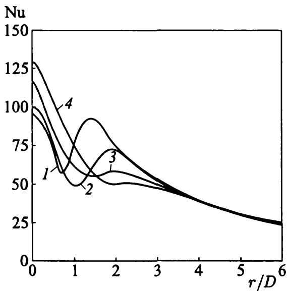
Рис. 5.48. Распределения числа Нуссельта по поверхности преграды при Re = 3 \cdot 10^4 и H/D = 1 (1); 2,5 (2); 5 (3); 8 (4)
