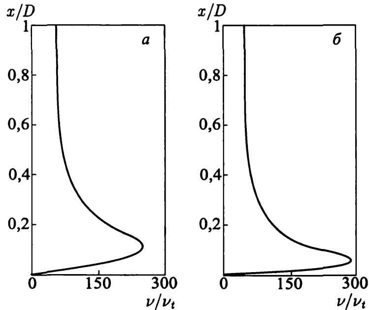
Рис. 5.47. Распределения турбулентной вязкости при H/D = 2 и Re = 2,3 \cdot 10^4 (фрагмент а); 7 \cdot 10^4 (фрагмент б)
