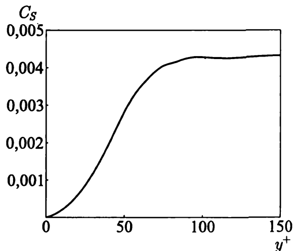
Рис. 5.8. Зависимость параметра Смагоринского от расстояния до стенки
