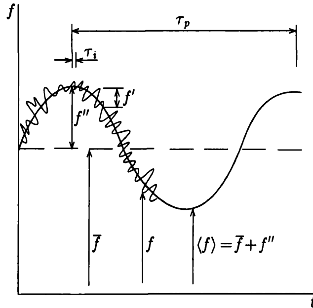
Рис. 2.1. Тройное разложение мгновенных значений параметров турбулентного потока
