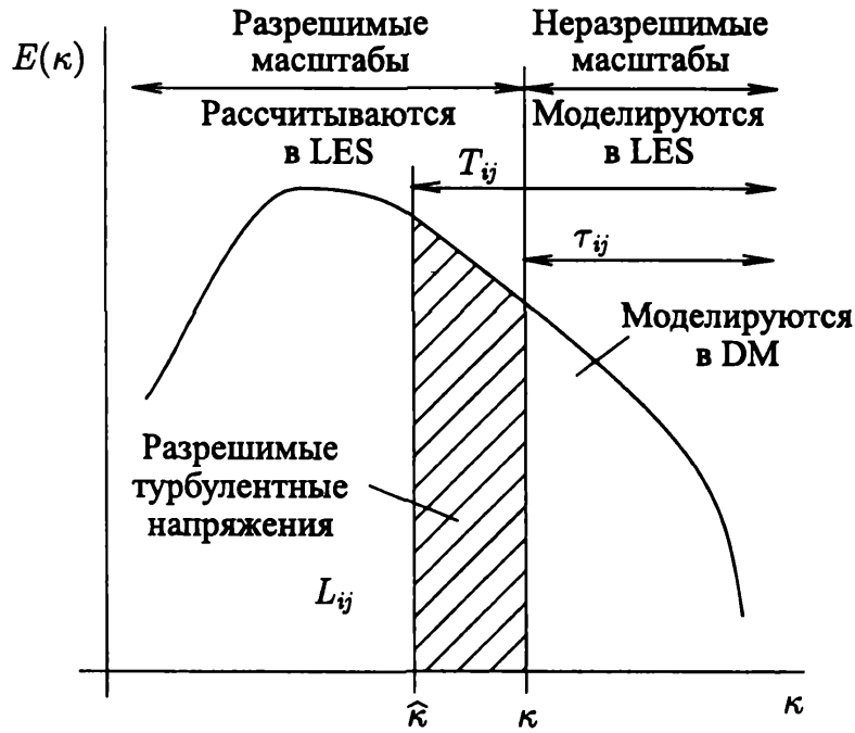
Рис. 3.2. Сеточный и тестовый фильтры в динамической модели
