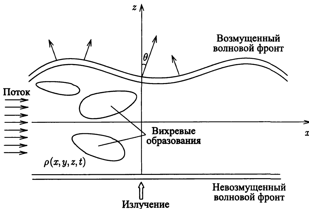
Рис. 5.58. Прохождение света через случайно-неоднородную среду
