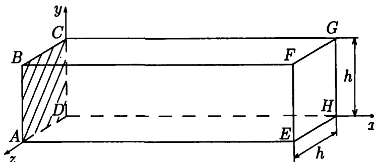
Рис. 5.9. Система координат
