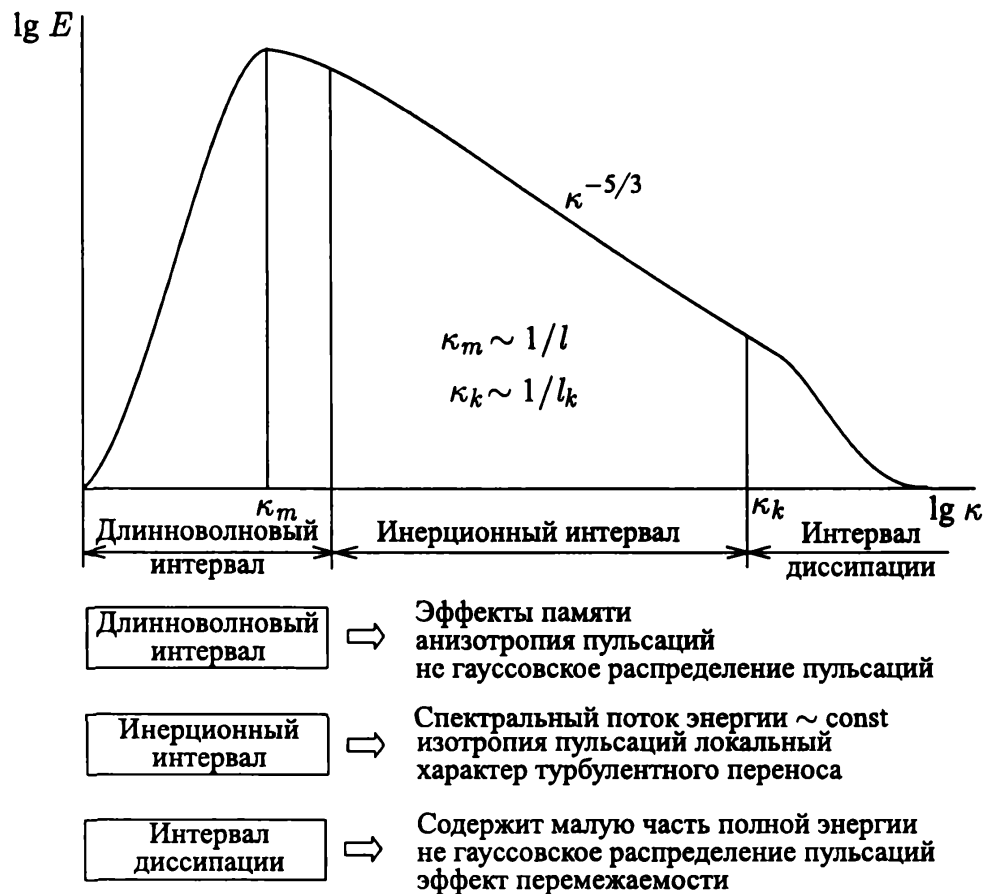
Рис. 1.1. Спектральная плотность кинетической энергии турбулентности
