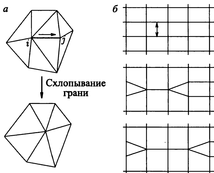
Рис. 4.9. Схлопывание ячейки в направлении наиболее короткой грани
