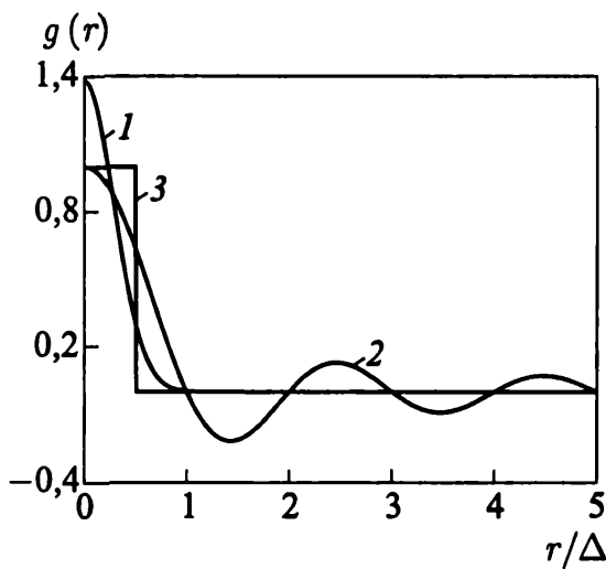
Рис. 2.3. Фильтрующие функции (1 — коробочный фильтр, 2 — гауссовский фильтр, 3 — Фурье-фильтр)
