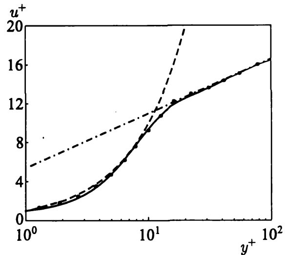
Рис. 5.3. Распределение скорости в пограничном слое
