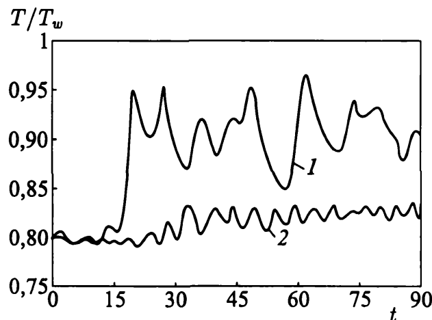
Рис. 5.52. Изменение температуры во времени на расстоянии x/D = 0,02 от поверхности преграды при H/D = 10 и Re = 10^3 . Кривые 1 и 2 соответствуют сечениям r = 0 и r = 4H
