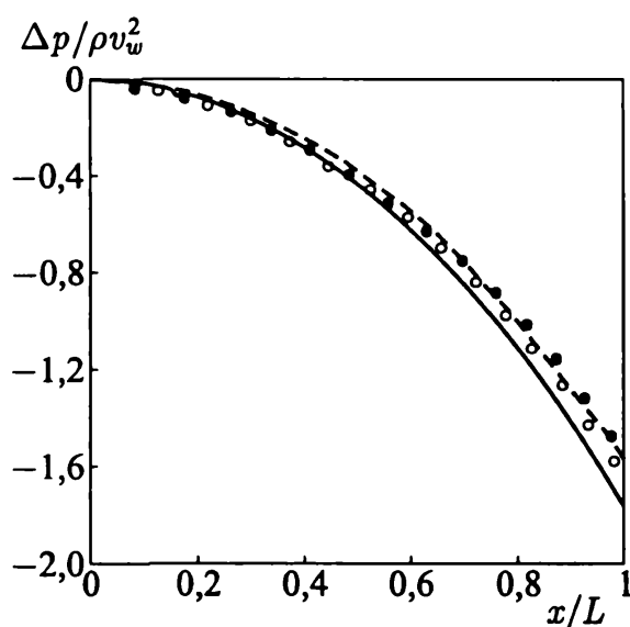
Рис. 5.17. Распределения давления в канале с двухсторонним вдувом при y/h = 0,5
