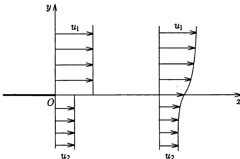
Рис. 5.23. Течение в слое смешения
