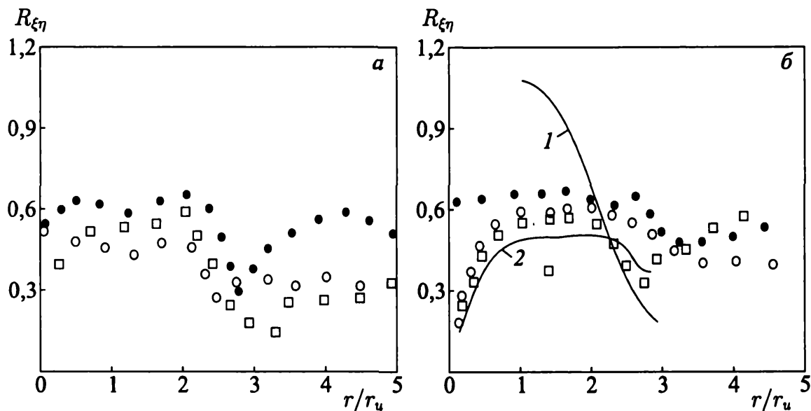
Рис. 5.39. Распределения корреляций осевой скорости и температуры (значки \bullet ), радиальной скорости и температуры (значки \circ ), осевой и радиальной скорости (значки \square ) при \vartheta = 2 в сечениях x/r_a = 10 (фрагмент а) и x/r_a = 30 (фрагмент б). Кривые 1 и 2 соответствуют данным [105] и [109]
