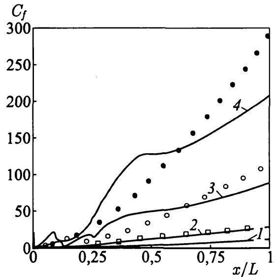
Рис. 5.16. Распределения коэффициента поверхностного трения вдоль непроницаемой стенки канала
