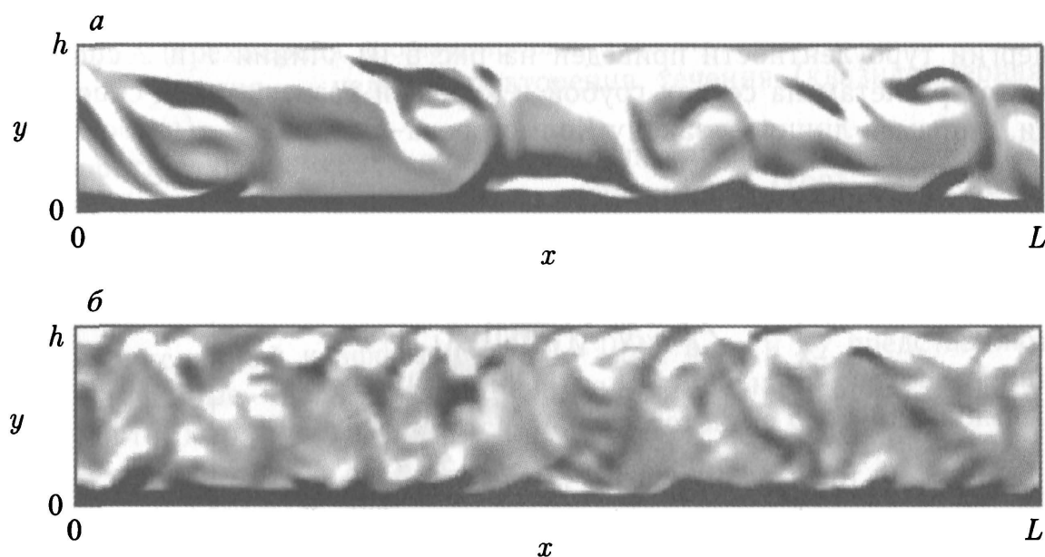
Рис. 5.12. Вихревая картина течения в канале при v_{w1} = 0 , v_{w2} = 1,0 м/с (фрагмент а) и v_{w1} = 0 , v_{w2} = 5,0 м/с (фрагмент б) в координатной плоскости xu
