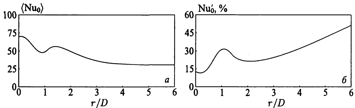
Рис. 5.55. Распределения среднего числа Нуссельта (фрагмент a ) и его флуктуаций (фрагмент б ) вдоль стенки при H/D = 1 и Re = 10^4
