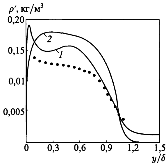
Рис. 5.59. Распределение флуктуаций плотности в пограничном слое. Кривая 1 соответствует результатам расчета, кривая 2 — расчету [318], значки • — данным измерений [318] (при M_c = 0,88 )
