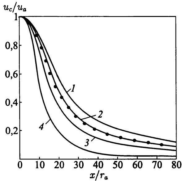
Рис. 5.33. Распределения осевой скорости вдоль оси струи при \vartheta = 0,6 (1); 1 (2); 1,8 (3). Кривая 4 соответствует данным [25] при \vartheta = 6 , значки \bullet — расчету по k-\epsilon модели [158]
