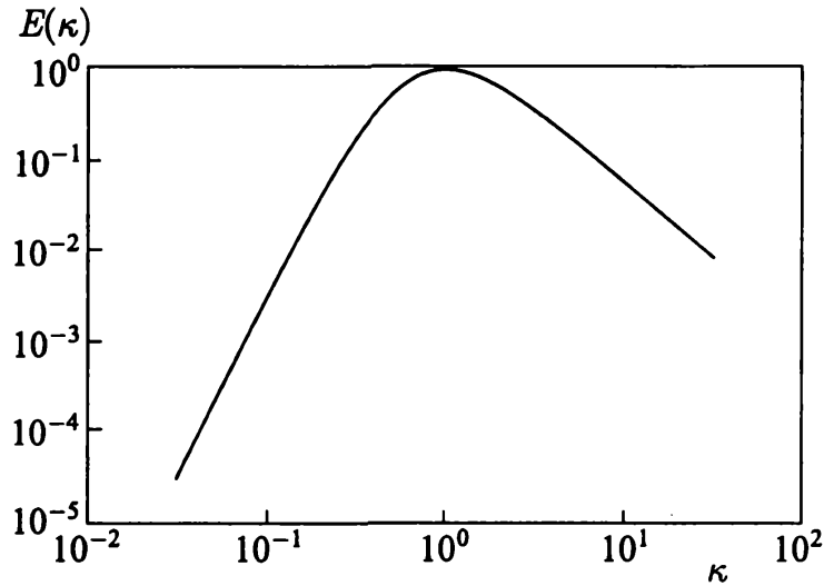
Рис. 1.2. Спектральная плотность кинетической энергии турбулентности, описываемая соотношением Кармана
