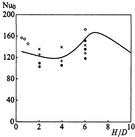
Рис. 5.50. Зависимость числа Нуссельта в точке торможения от относительного расстояния от среза сопла до преграды при Re = 2,3 \cdot 10^4 . Сплошная линия соответствует результатам расчета, значки \bullet — данным [69, 70]; \circ — данным [230]; \times — расчету по k - \epsilon модели [328]; + — расчету по SST-модели [328]
