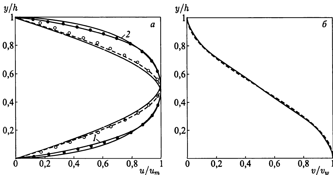
Рис. 5.14. Распределения продольной (фрагмент а) и поперечной (фрагмент б) скорости при v_{w1} = v_{w2} = 2,75 м/с и x/h = 20 (1); 60 (2)
