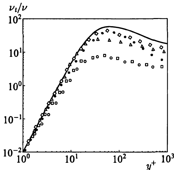
Рис. 5.7. Распределение турбулентной вязкости около стенки
