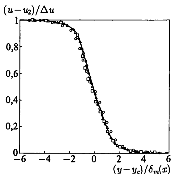
Рис. 5.24. Профили продольной скорости и сравнение моделей подсеточной вязкости
