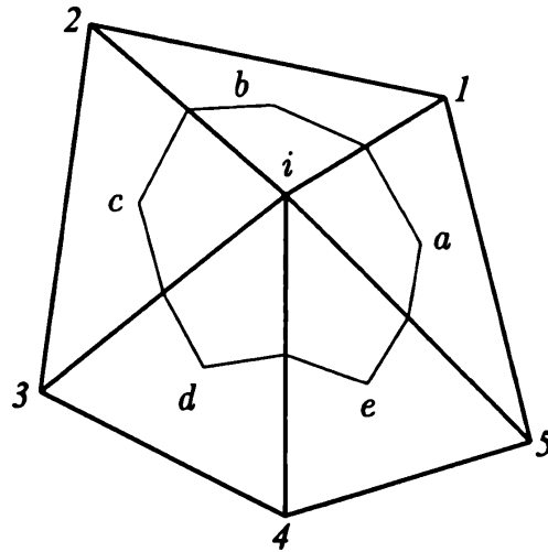
Рис. 4.7. Вычисление градиента
