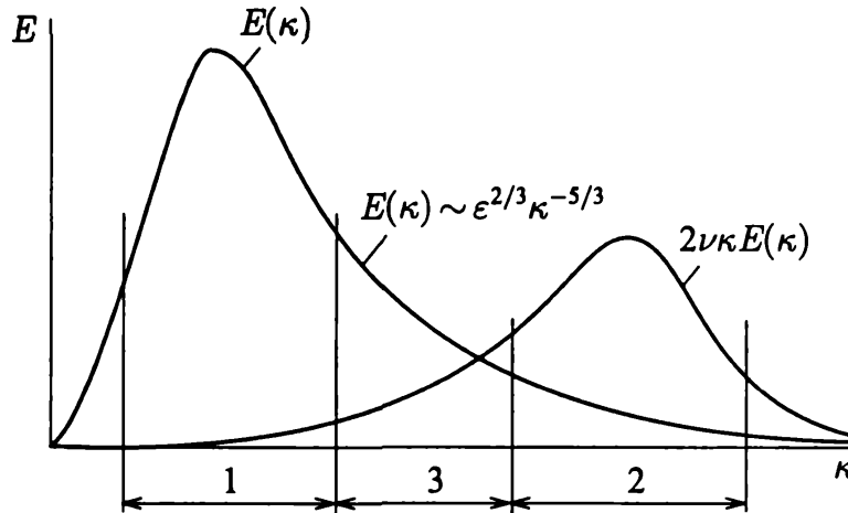
Рис. 1.3. Интервал энергии (участок 1), интервал диссипации (участок 2) и инерционный интервал (участок 3)
