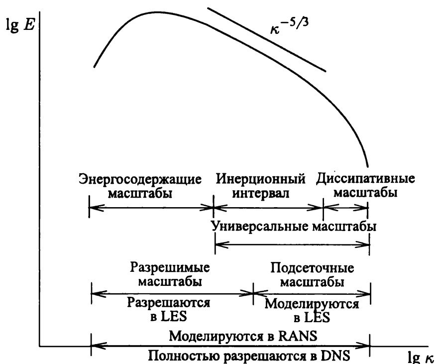
Рис. 1.5. Спектр кинетической энергии турбулентности и трактовка различных подходов к моделированию турбулентных течений
