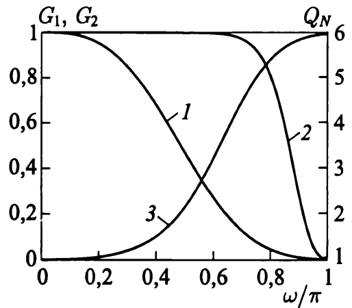
Рис. 3.5. Явный фильтр на равномерной сетке G (кривая 1), фильтр \hat{G}_2 (кривая 2), \hat{Q}_N при N = 5 (кривая 3)
