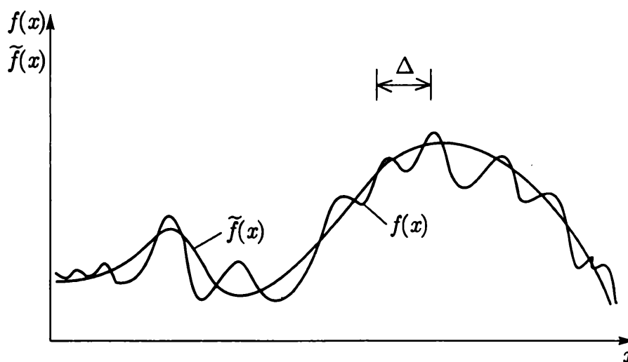
Рис. 1.8. Исключение мелкомасштабных пульсаций при помощи фильтрации
