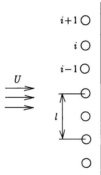
Рис. 4.11. Внесение возмущений
