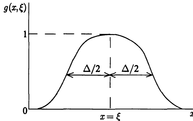
Рис. 2.2. Фильтрующая функция
