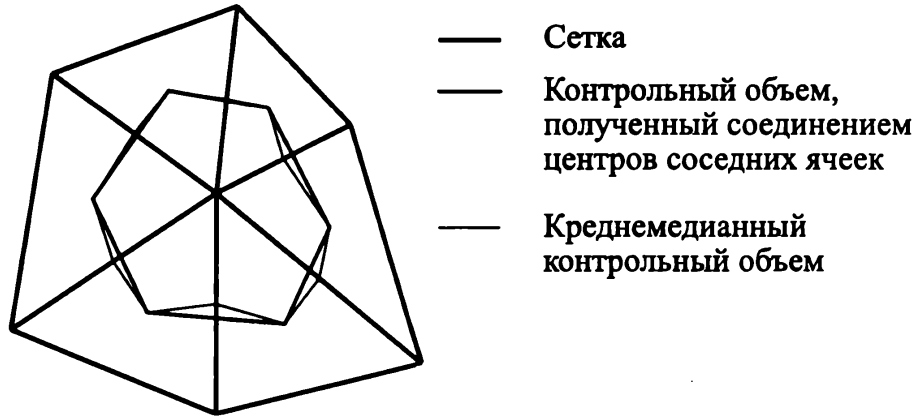
Рис. 4.6. Среднемедианный контрольный объем
