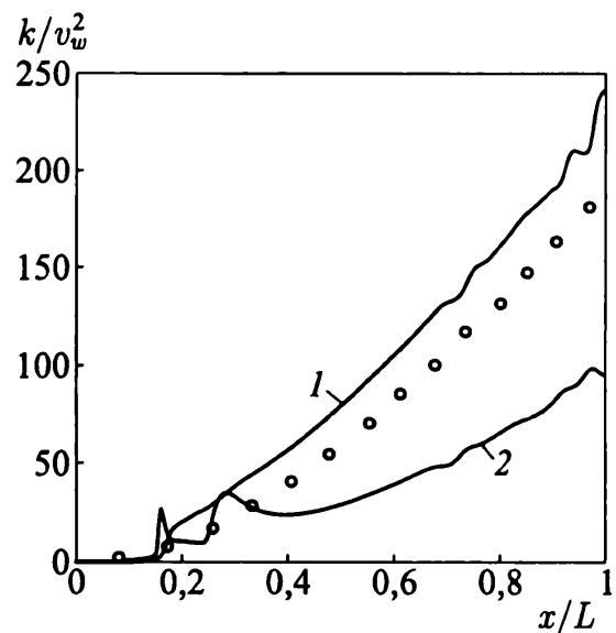
Рис. 5.19. Распределения кинетической энергии турбулентности при y/h = 0,5 (1); 0,75 (2)
