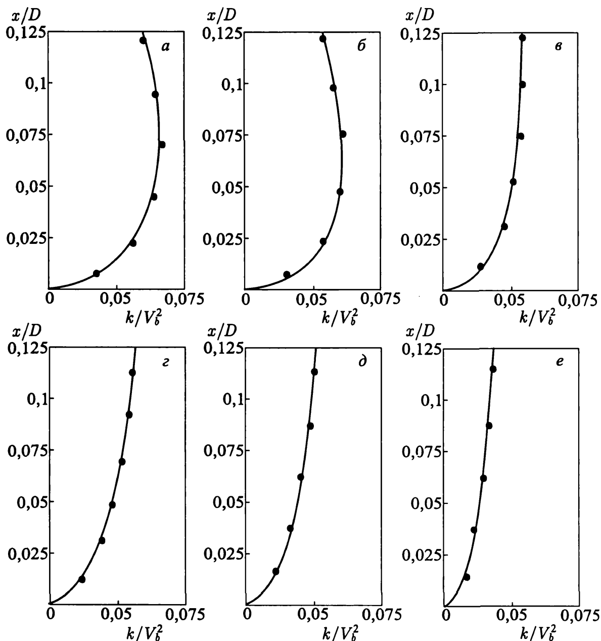
Рис. 5.46. Распределения кинетической энергии турбулентности в сечениях r/D = 0,5 (а); 1 (б); 1,5 (в); 2 (г); 2,5 (д); 3 (е) при H/D = 4 и Re = 7,0 \cdot 10^4 . Значки • соответствуют данным измерений [69, 70]
