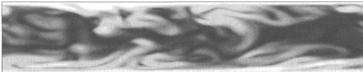
Рис. 5.1. Вихревая картина течения в канале при t = 0,32 \text{ с}
