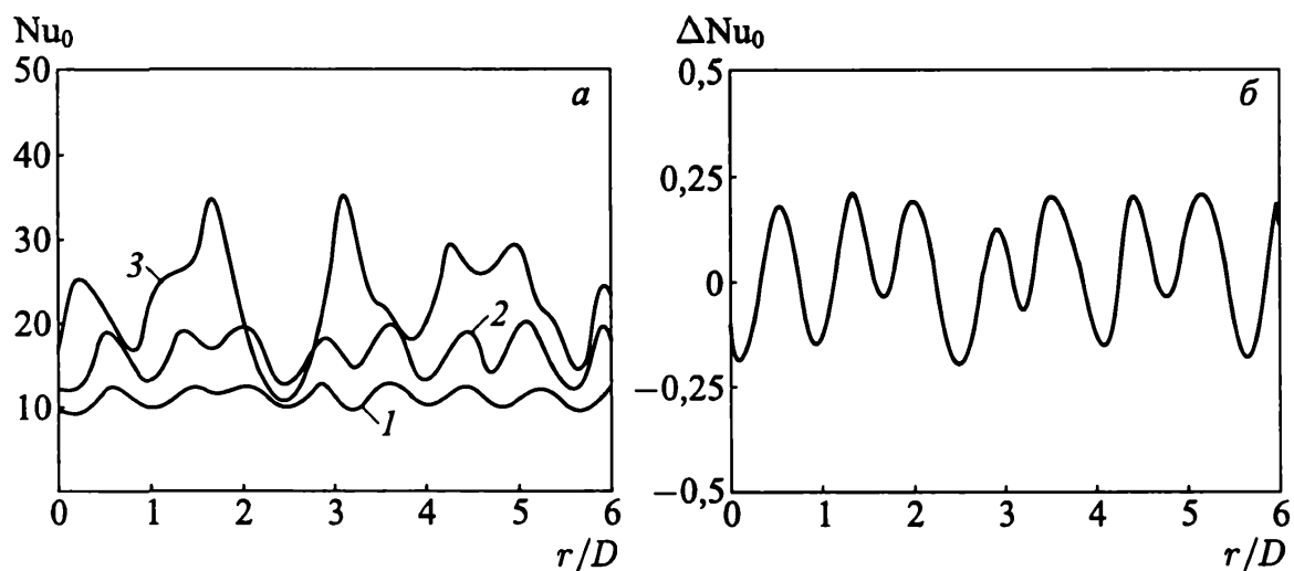
Рис. 5.54. Зависимость числа Нуссельта в точке торможения от времени (фрагмент a ) и его отклонение от среднего значения (фрагмент б ) при H/D = 5 . Кривые 1, 2, 3 на фрагмент a соответствуют значениям Re = 300, 500, 1000 , а кривая на фрагмент б — Re = 500
