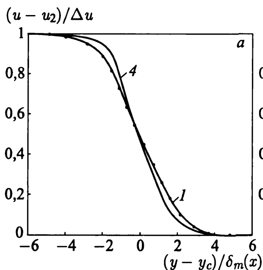
Рис. 5.26. Профили продольной (фрагмент а) и поперечной (фрагмент б) скорости при M_c = 0,2 (1); 0,4 (2); 0,6 (3); 0,8 (4). Значки \bullet соответствуют расчетным данным [148]
