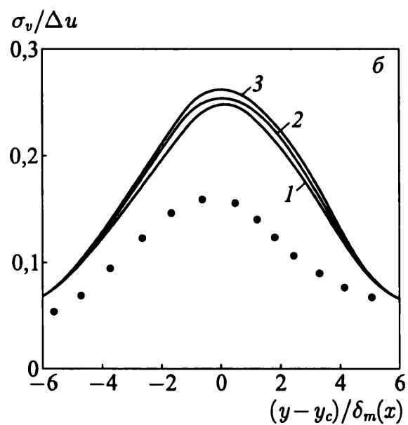
Рис. 5.28. Распределения интенсивности пульсаций продольной (фрагмент а) и поперечной (фрагмент б) скорости в сравнении с экспериментальными данными [169] (значки \bullet ) при x/L_x = 0,6 (1); 0,7 (2); 0,8 (3)
